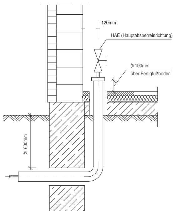
Schnitt A-A
