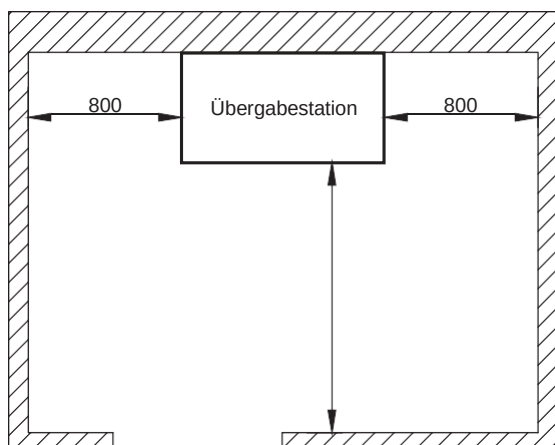
Abbildung 7.4.3 Platzbedarf für Übergabestationen
