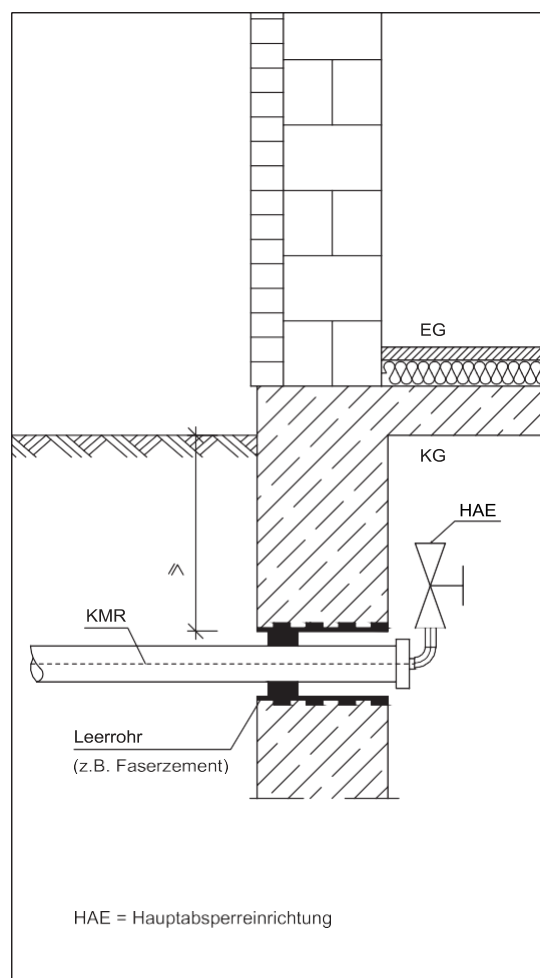
Unterkellerte Gebäude
