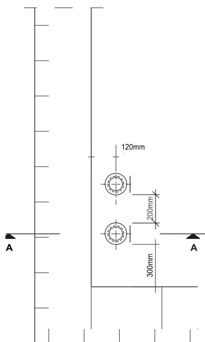
Draufsicht
