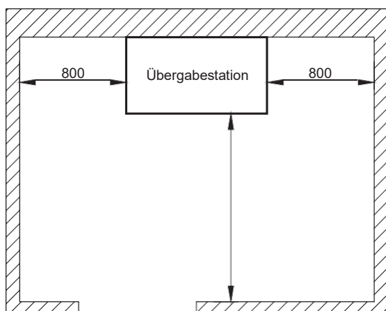
Abbildung 7.5.3 Platzbedarf für Übergabestationen
