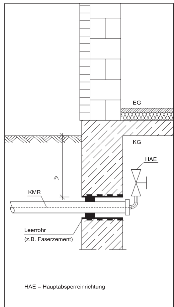
Unterkellerte Gebäude
