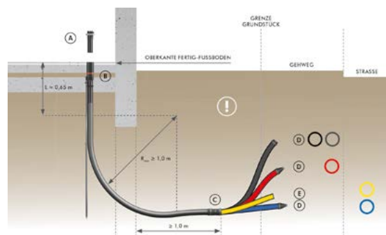
Abbildung: Einbauhinweis QS Basic R4+
