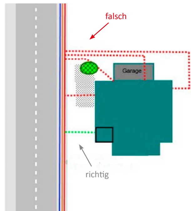
Abbildung: Lageplan Hausanschlussstrasse
