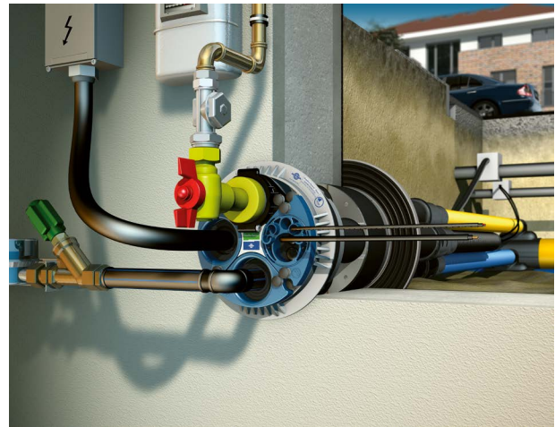
Abbildung: Quadro-Sicura 1 Nova
