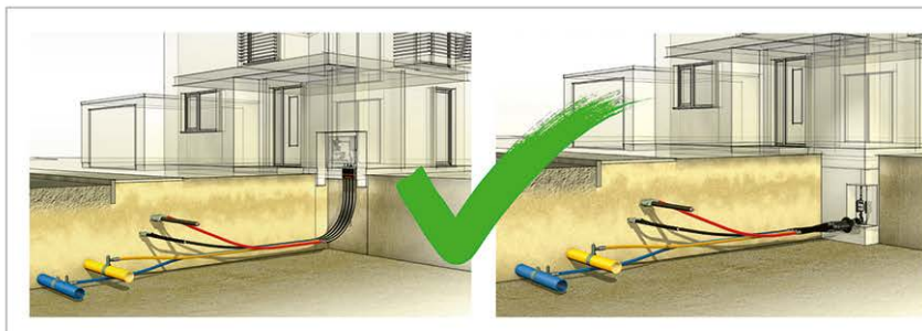
Abbildung: Beispiel einer normgerechten Ausführung
